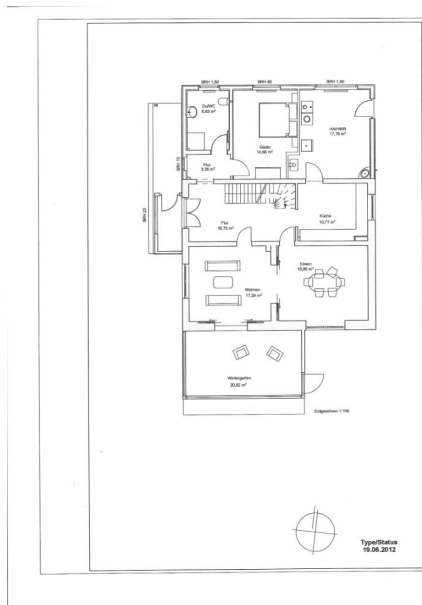
Grundriss Erdgeschoss
