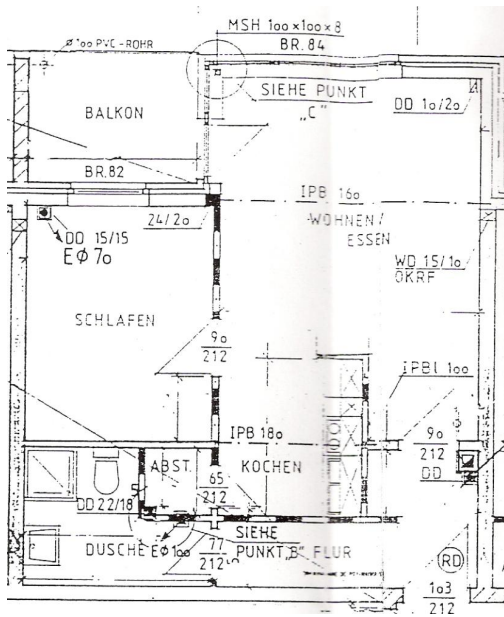
Grundriss
